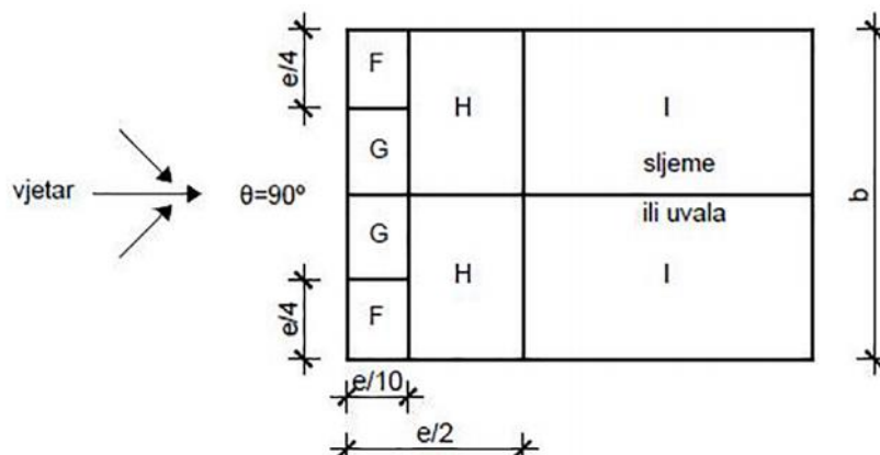
Slika 6. Podjela krovne plohe na zone djelovanja vjetra [2]
