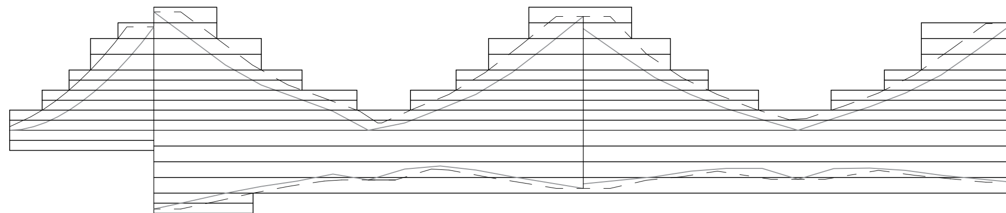
F_{Sd} DIJAGRAM 1cm = 300 kN
