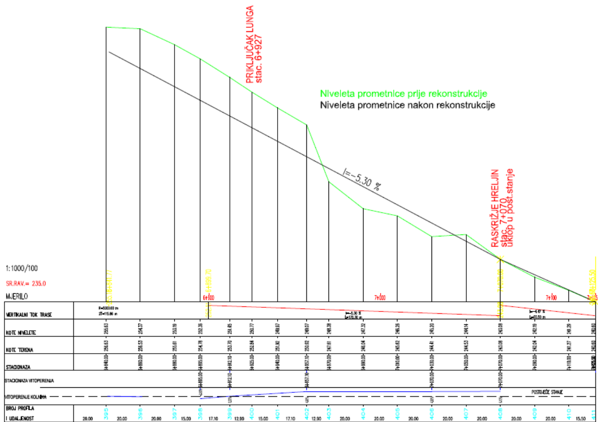
Slika 49: Uzdužni presjek stare i nove nivelete prometnice (izradio autor)
