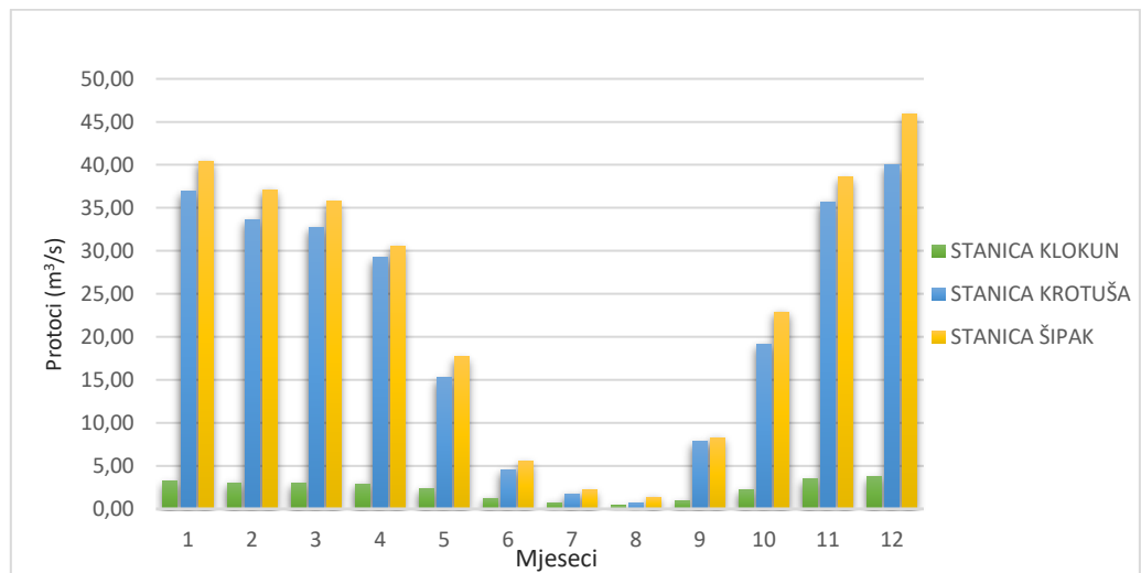
Slika 34. Grafički prikaz srednjih vrijednosti godišnjih nizova na mjernim postajama Baćina, Krotuša i Šipak (razdoblje 1979-2020.) za maksimalne protoke: (izradio autor)
