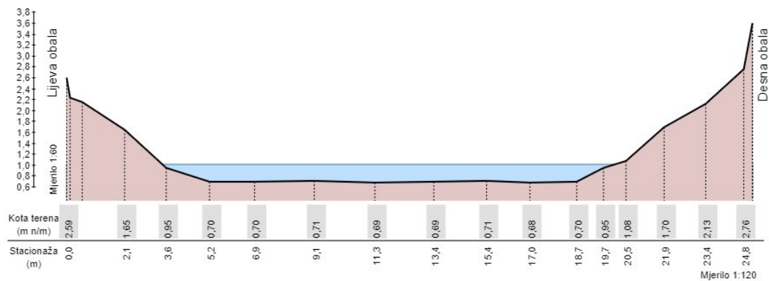
Slika 29. Poprečni presjek korita na mjerne postaji Šipak; preuzeto sa: ( https://hidro.dhz.hr/ )
