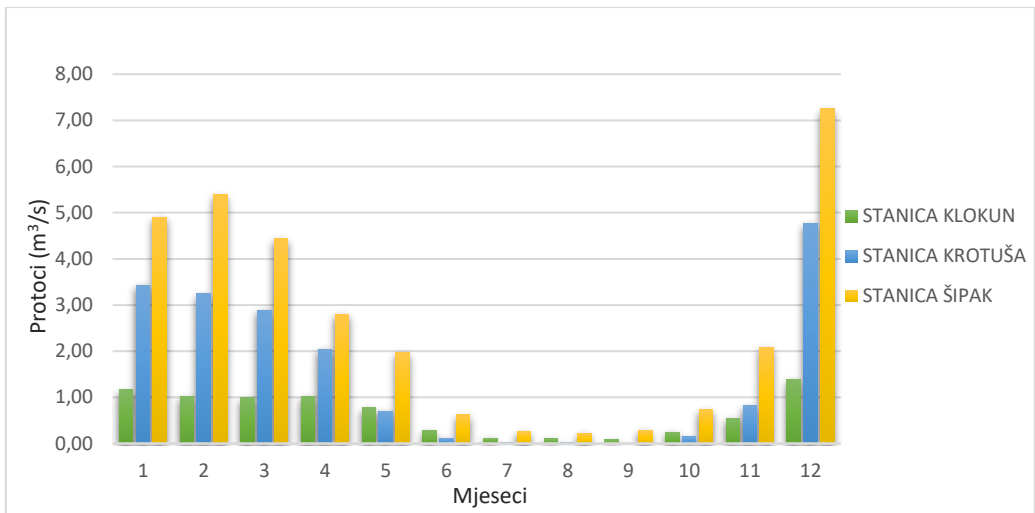
Slika 32. Grafički prikaz srednjih vrijednosti godišnjih nizova na mjernim postajama Baćina, Krotuša i Šipak (razdoblje 1979-2020.) za minimalne protoke: (izradio autor)
