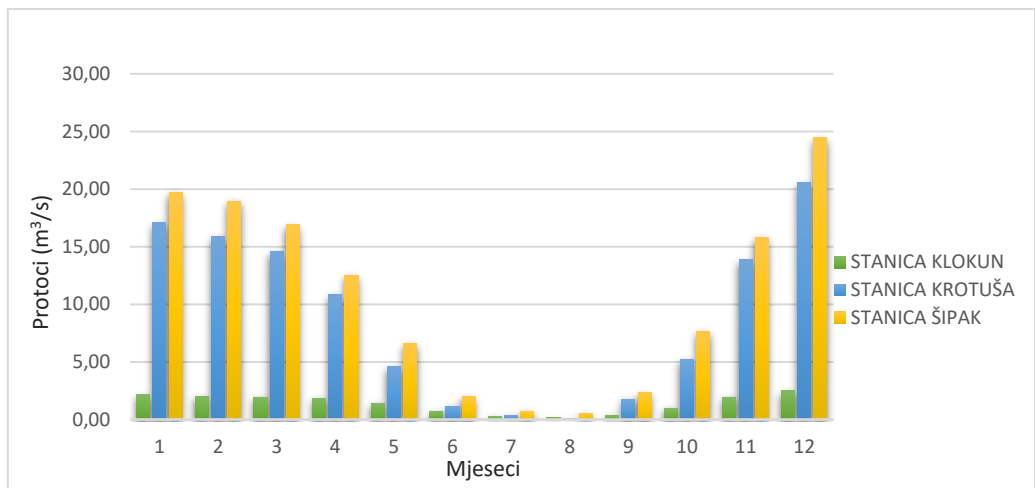
Slika 33. Grafički prikaz srednjih vrijednosti godišnjih nizova na mjernim postajama Baćina, Krotuša i Šipak (razdoblje 1979-2020.) za srednje protoke: (izradio autor)
