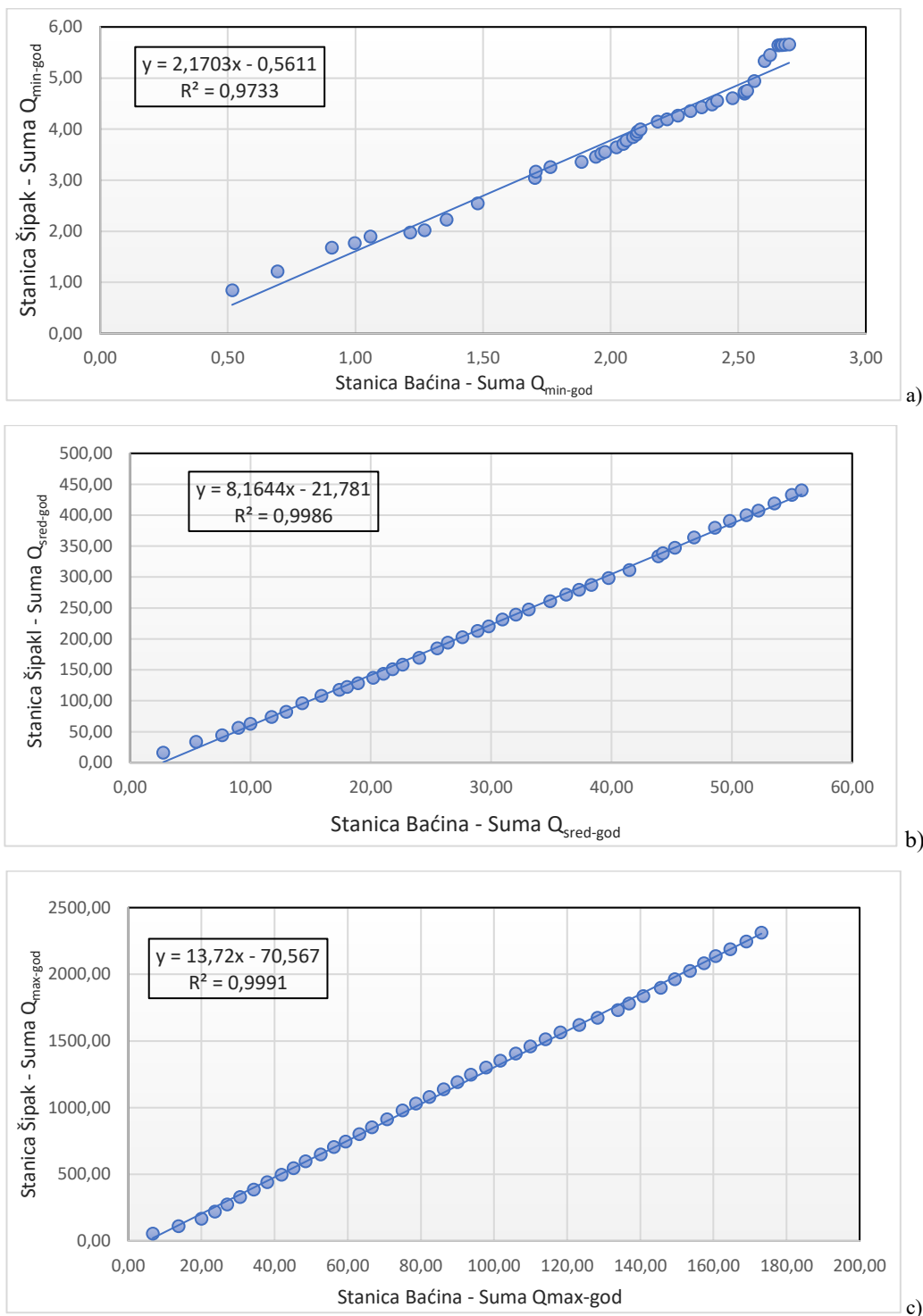
Slika 42. Mjerne postaje Baćina i Šipak - analiza homogenosti za minimalne (a) , srednje (b) i maksimalne (c) protoke za razdoblje od 1979. do 2020. god.: (izradio autor)
