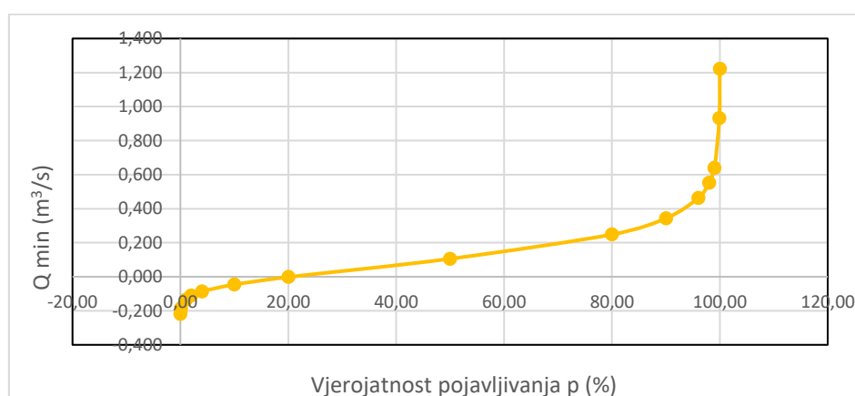
Slika 44. Grafički prikaz vjerojatnosti pojave minimalnih godišnjih protoka u smjeru najmanjih vrijednosti na mjernoj postaji Šipak za razdoblje od 1979. do 2020. god.: (izradio autor)
