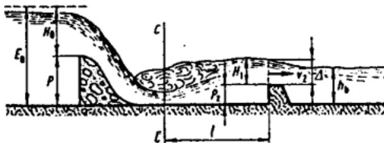
Slika 21. Poduprt skok ispred zida (Agroskin, 1969.)
