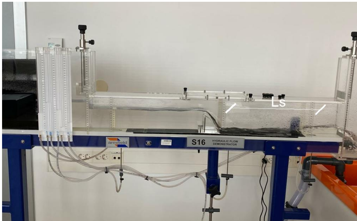
Slika 9. Određivanje duljine vodnog skoka u laboratoriju
