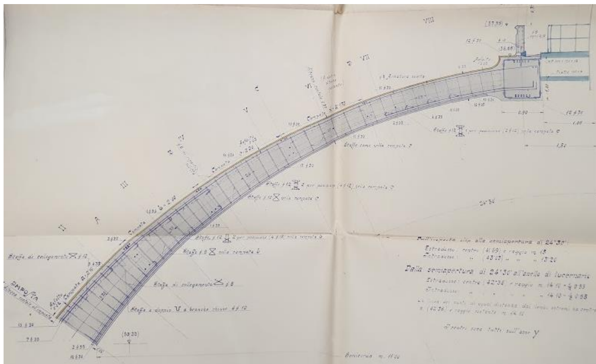
Slika 33: Kupola Gina Veronesea – presjek kroz rebro (meridijan) [4]
