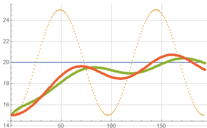
Dijagram 21: Prikaz promjene temperatura na plohami troslojnog stakla
