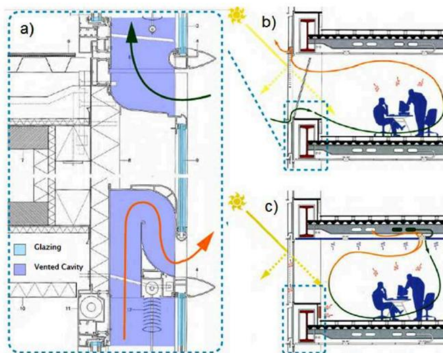
Slika 21. Detalj ventilacije
