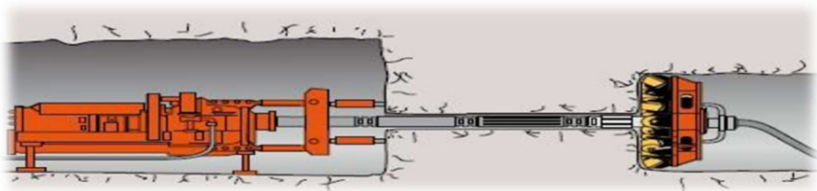
Slika 18 : Bušenje mikrotunela [5]
