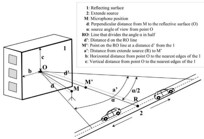
Slika 7: Mikrofon u blizini reflektirajuće površine [10]
