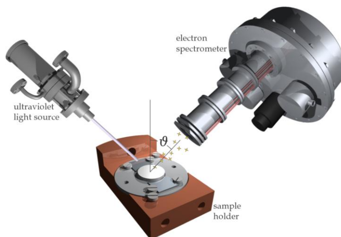
Slika 14 Eksperiment kutno razlučne fotoemisije spektroskopije (ARPES). Žarulja s izbojem helija obasjava ultraljubičasto svjetlo na uzorak u ultra visokom vakuumu. Hemisferični analizator elektrona mjeri distribuciju izbačenih elektrona s obzirom na energiju i moment. [10]
