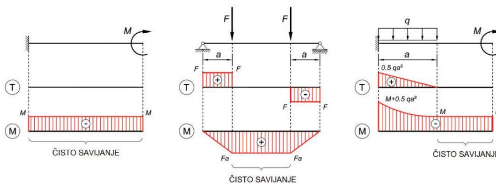
Slika 1: Čisto savijanje [3]
