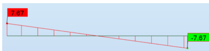
Slika 27. Vrijednost poprečne sile V_z podrožnice. Za kombinaciju 113
