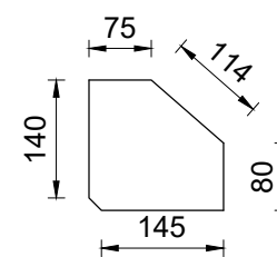
DIMENZIJE UKRUTE
