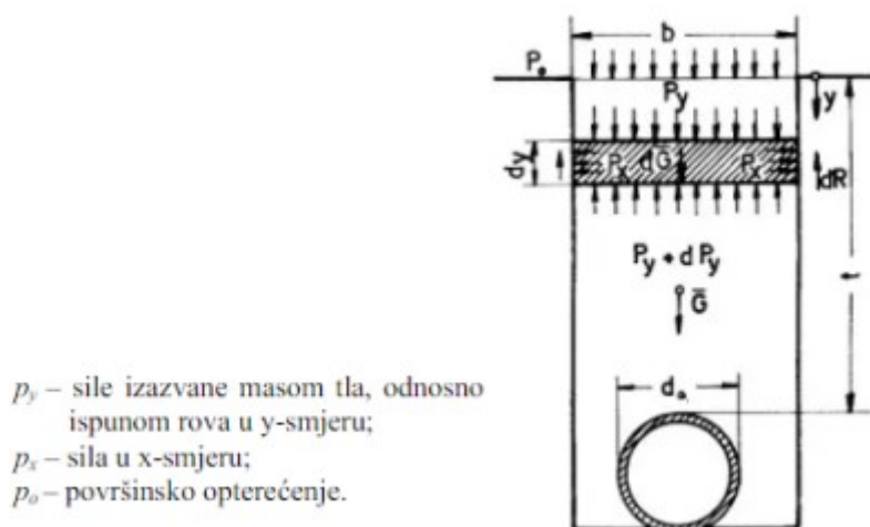
Slika 38. Raspored sila u rovu [3]
