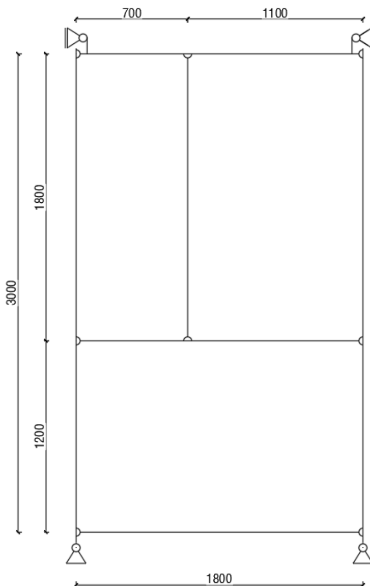
Slika 17. Statički sustav fasadnog elementa
