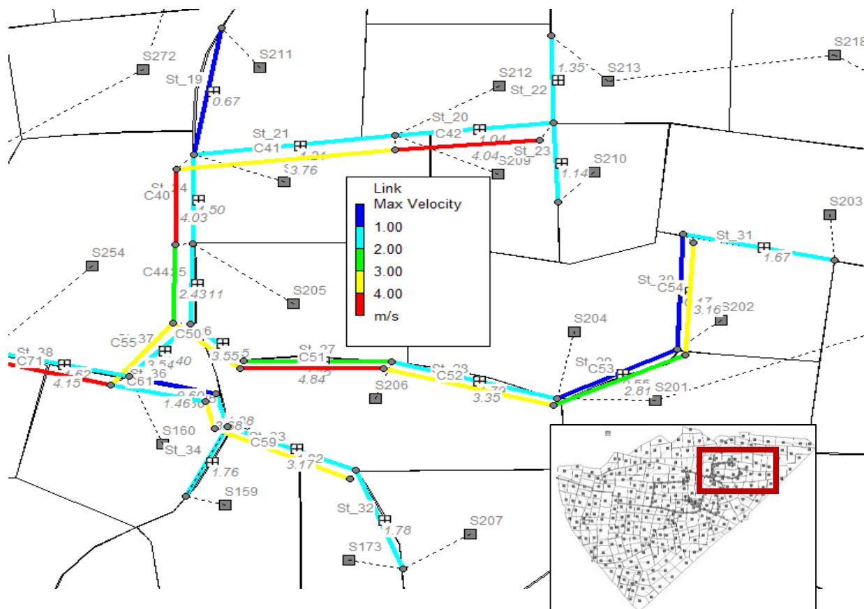
Slika 78. Grafički prikaz maksimalnih brzina u cijevima u podstava 1 za sadašnje stanje (PP 100.god., 3h)
