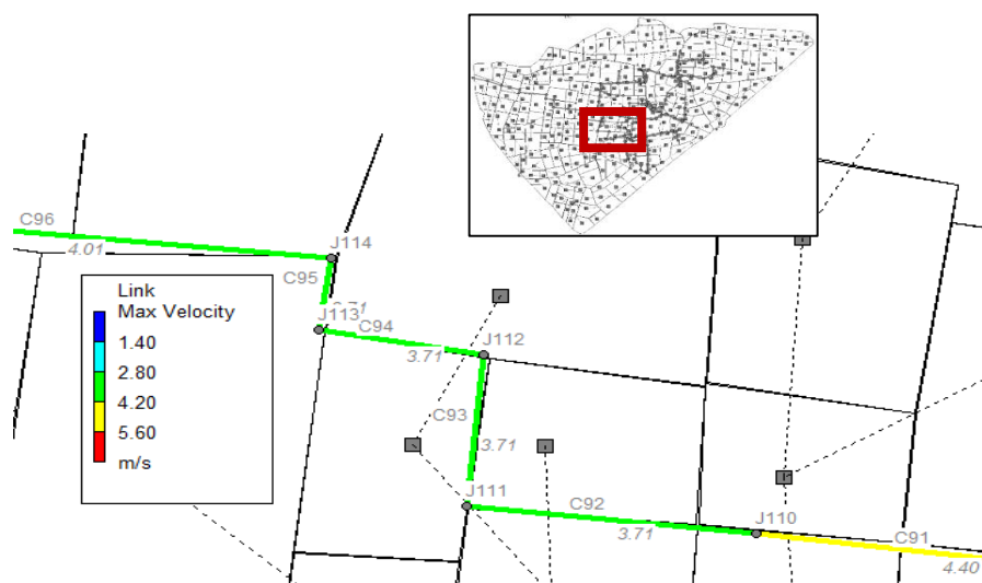
Slika 126. Grafički prikaz maksimalnih brzina u cijevima u podsustavu 9 za buduće stanje (PP 25 god., 3h)
