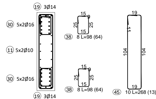
Presjek 10-10 MJ. 1:25
