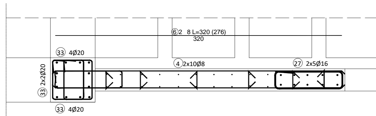
Presjek 6-6 MJ. 1:25
