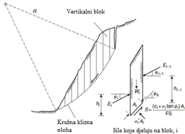
Slika 18. Tipični rotacijski slom; kružna ploha velikog radijusa u homogenoj slaboj stijeni [2]
