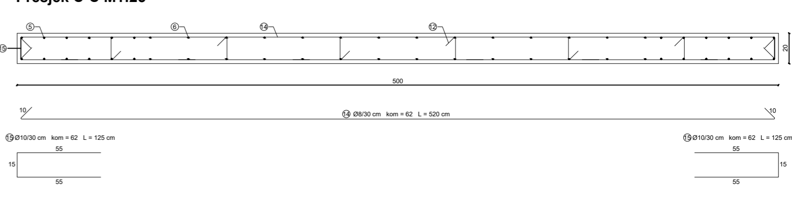
Presjek C-C M1:25
