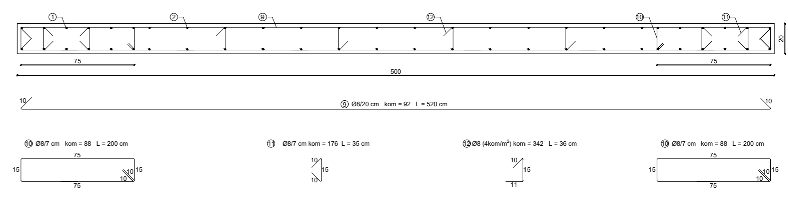
Presjek A-A M1:25
