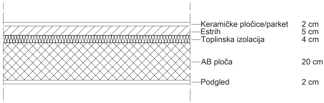
Slika 5. Slojevi ploča zgrade
