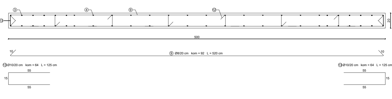
Presjek B-B M1:25
