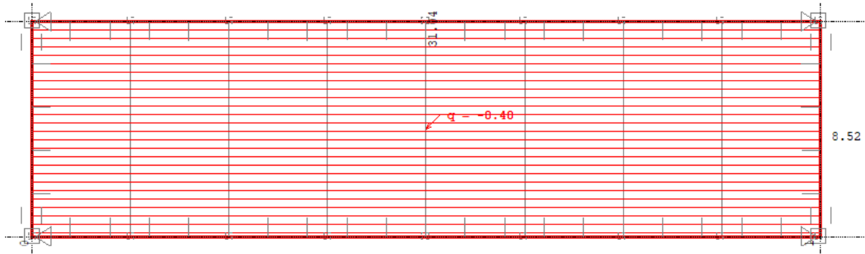
Slika 27. Prikaz opterećenja od snijega u tlocrtu [kN/m 2 ]
