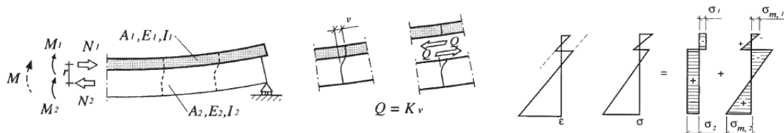
b) Raspodjela unutrašnjih sila i posmična ravnina spoja
