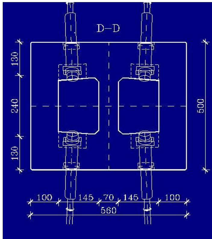
Slika 9: Presjek R4
