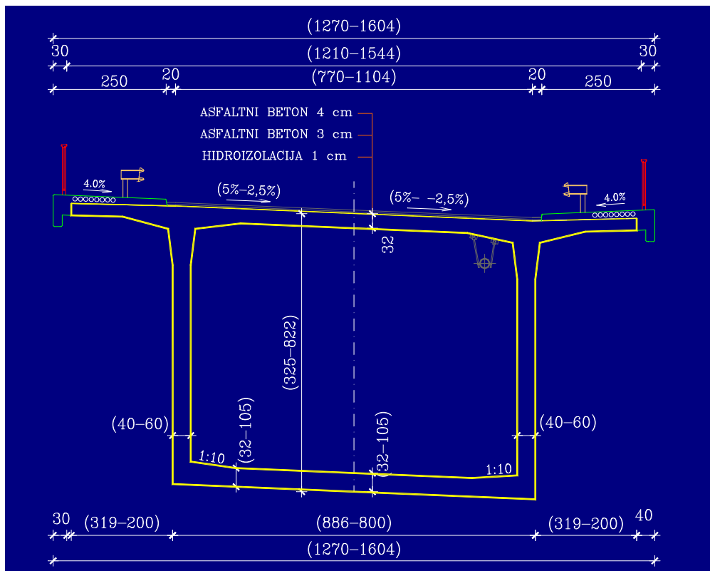
Slika 10: Presjek R5 i R6
