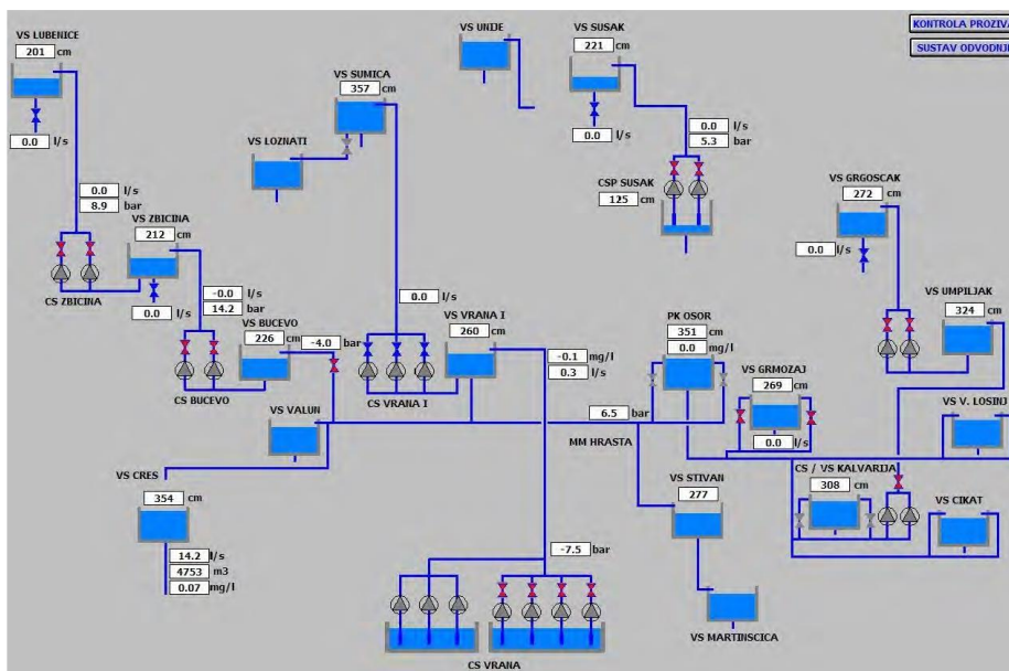
Slika 2.11. Shematski prikaz današnjeg vodoopskrbnog sustava otoka Cresa i Lošinja (Institut IGH, 2016,)
