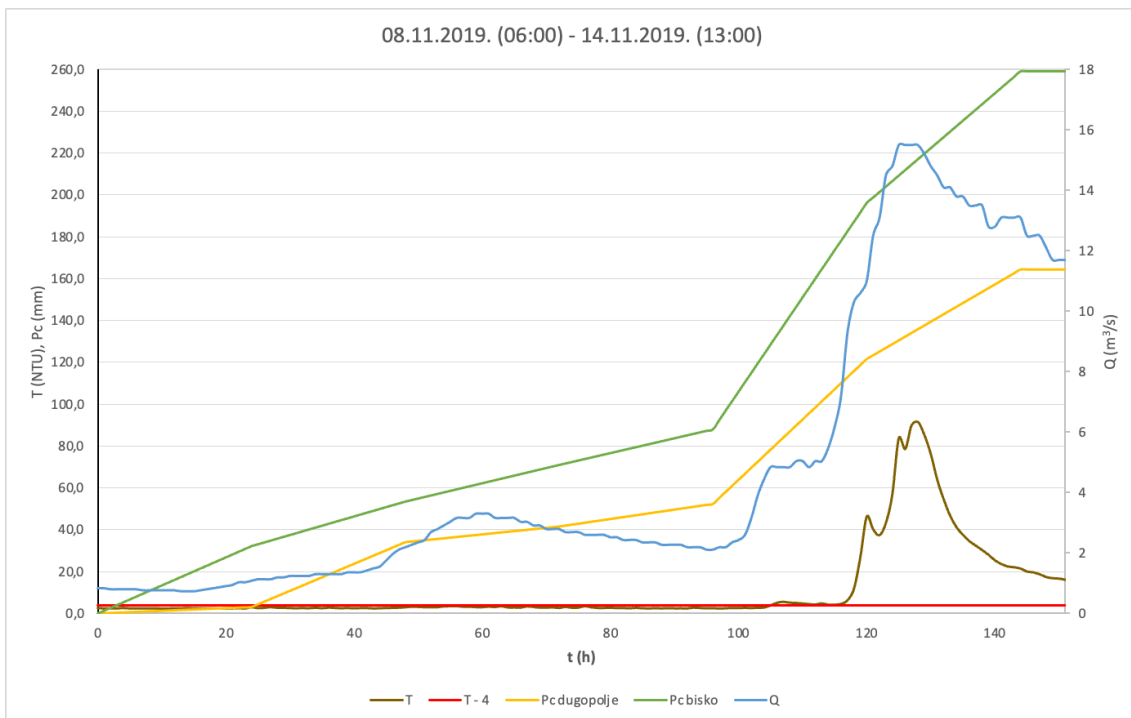
Slika 70: Prikaz vremenskih nizova satne mutnoće (T), protoka (Q) i kumulativne količine oborina za oborinske događaje s prekoračenjem mutnoće u 2019., s datumima početka i završetka svakog događaja. (izradio autor);
