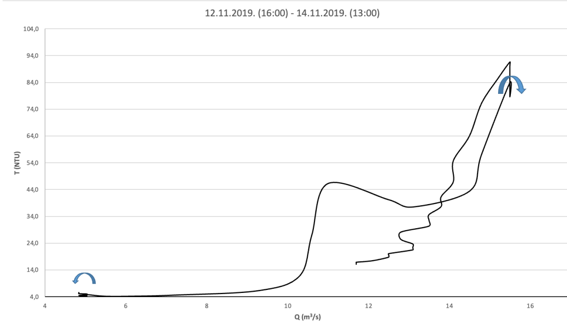
Slika 71: Prikaz dijagrama histereze prekoračenja mutnoće (Te) u odnosu na protok (Q) (Te-Q) za događaj 12.. Dominantni smjerovi histereze označeni su strelicama. (izradio autor);
