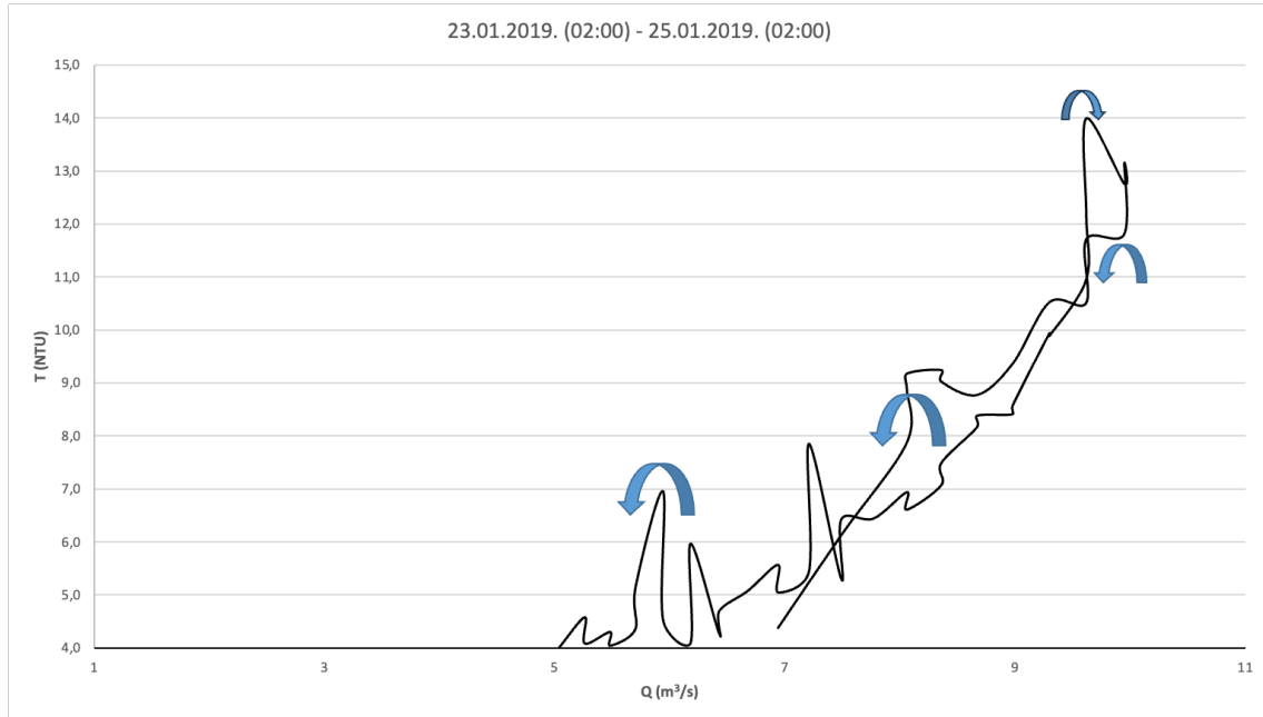
Slika 65: Prikaz dijagrama histereze prekoračenja mutnoće ( T_e ) u odnosu na protok ( Q ) ( T_e - Q ) za događaj 9. Dominantni smjerovi histereze označeni su strelicama. (izradió autor);
