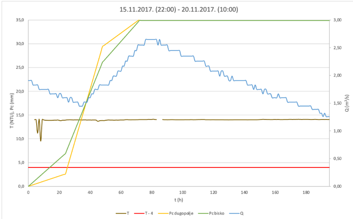
Slika 55: Prikaz vremenskih nizova satne mutnoće ( T ), protoka ( Q ) i kumulativne količine oborina za oborinske događaje s prekoračenjem mutnoće u 2017., s datumima početka i završetka svakog događaja. (izradio autor);
