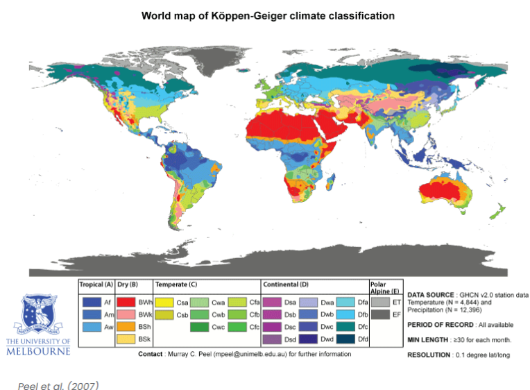
Slika 20. Koppen-Geiber klasifikacija [26]
