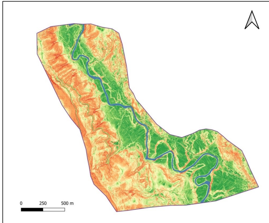
Slika 15: Karta nagiba pilot područja u udolini Rječine izvedena iz DMR-a: zelena boja – ravni dijelovi terena, smeđa boja – strmi nagibi padina.
