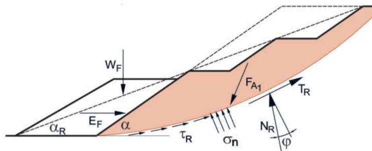
Slika 11. Smanjenje općeg nagiba kosine [17]
