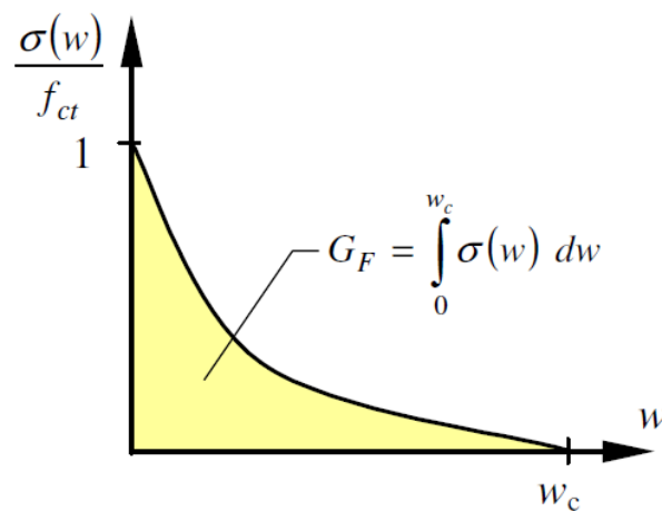
Slika 5.2 Dijagram naprezanje u betonu - širina pukotine ( \sigma-w ) [29]
