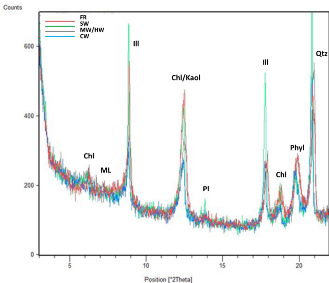
Slika 4.78 Difrakcijske slike neorijentiranih frakcija čestica < 2 μm uzorka flišne stijenske mase različitih stupnjeva trošnosti iz doline Rječine u području niskih kuteva 2θ (područje razlikovanja pojedinih minerala glina)
