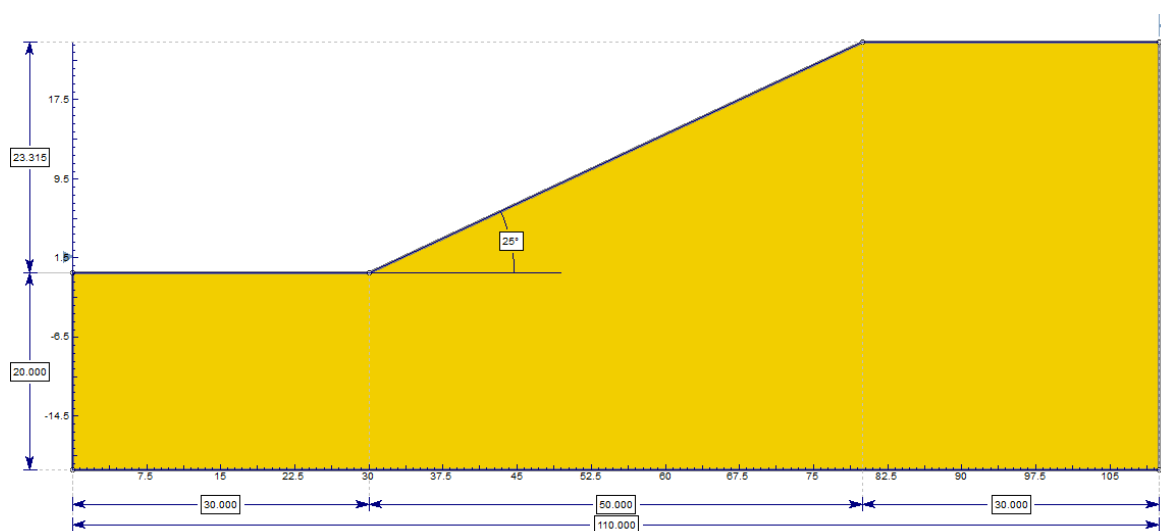
Slika 19: Geometrija modela kosine
