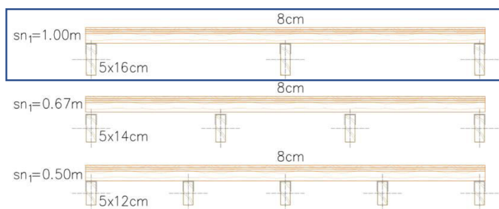
Slika 42: Most širine 2.0m – opterećenje pješacima – mogući statički slučajevi
