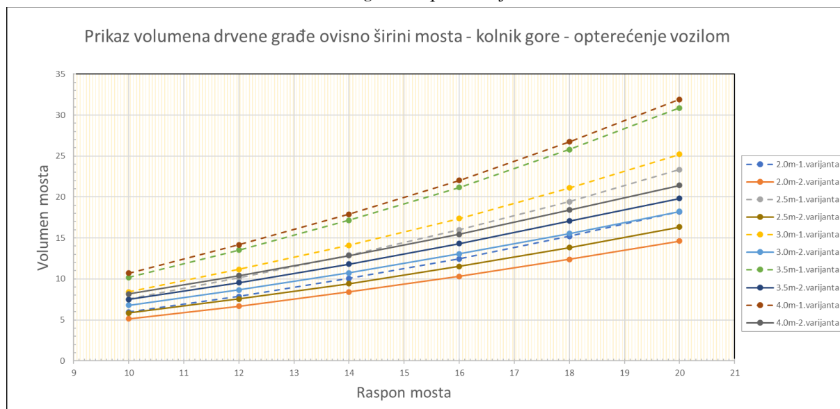
Graf 33: Prikaz ukupnog volumena drvene građe ovisno o rasponu i širini mosta – varijante mosta sa kolnikom gore – opterećenje vozilo
