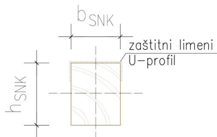
Slika 37: Karakteristični presjek sekundarne uzdužne grede
