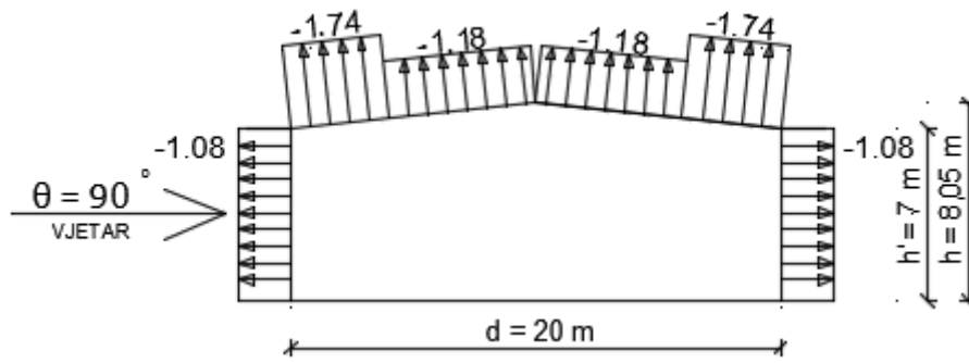
Slika 12.1. Presjek 1 - 1
