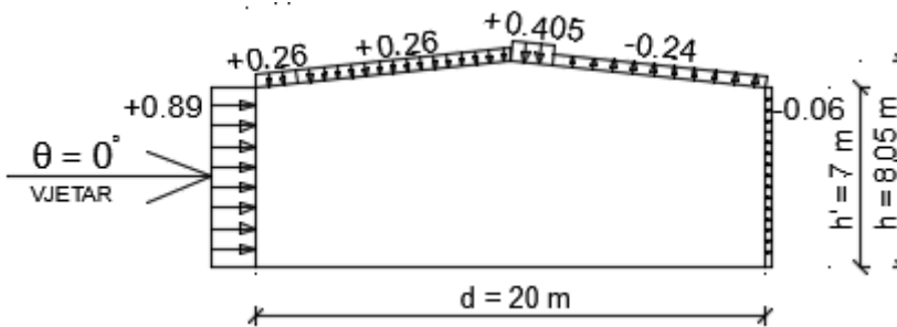
Slika 9.3. Presjek 1 - 1 [2]
