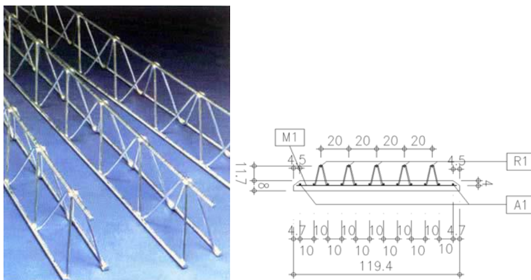
Slika 15: Prikaz R-nosača [11]
