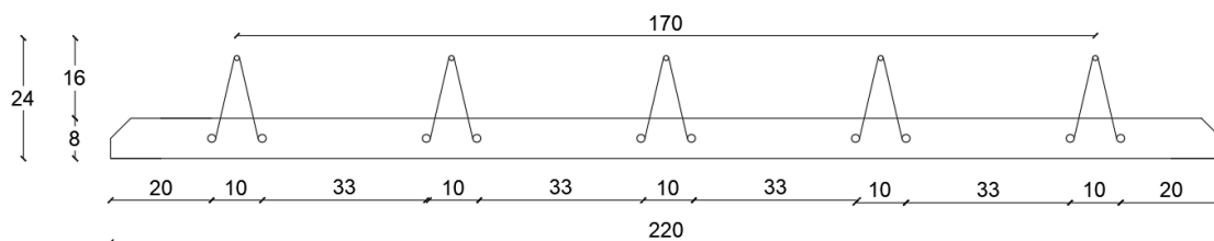
Slika 17: Poprečni presjek omnia ploče
