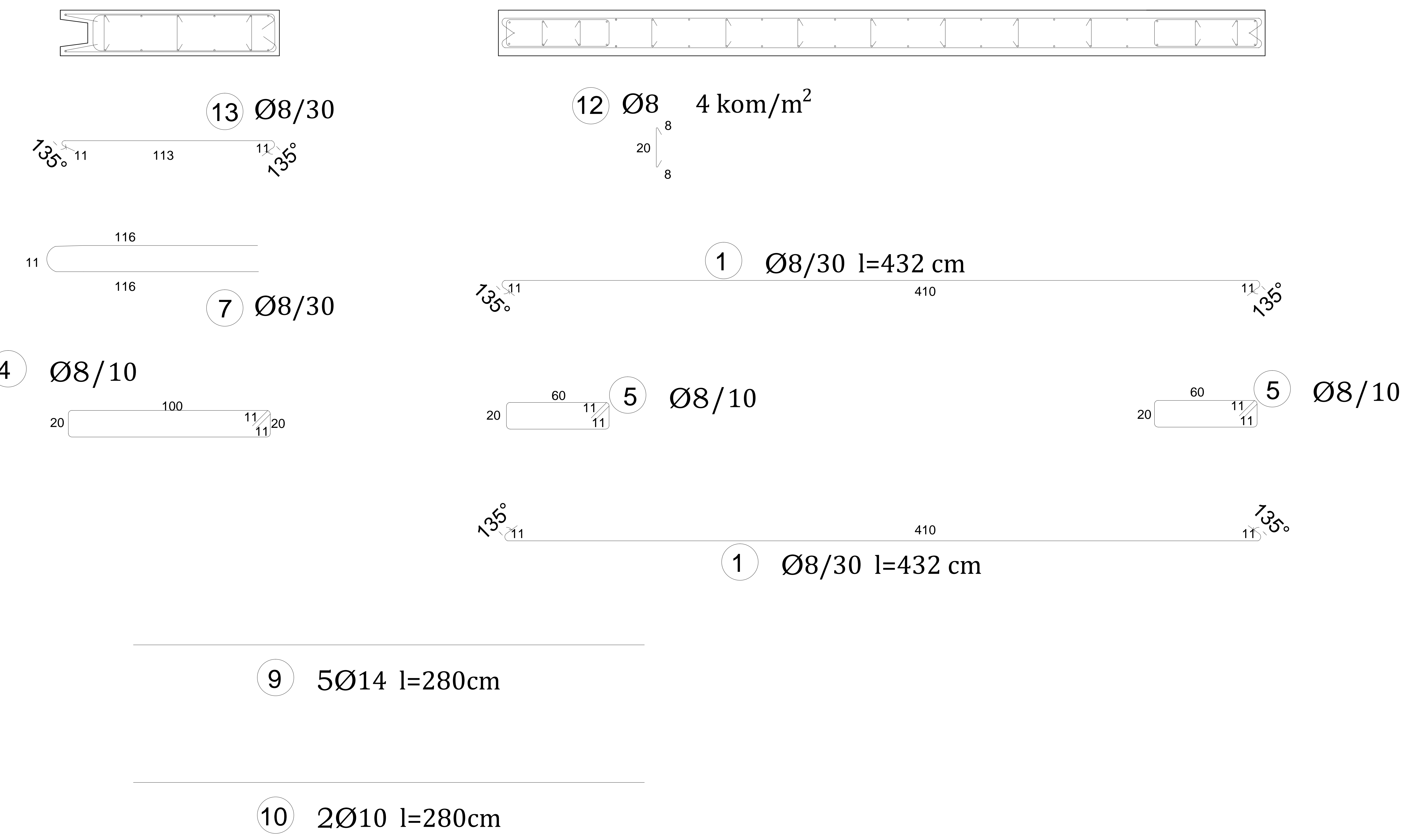
Presjek 1-1
