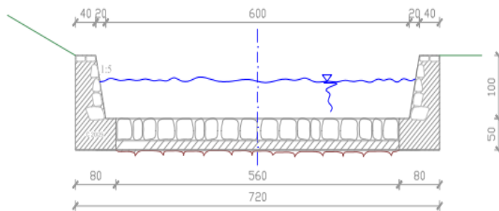
c) NORMALNI PROFIL KANALA OD 0+102,76 DO 0+122,40
