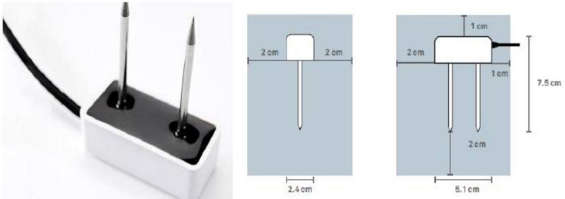
Slika 20: Senzor TEROS 10 [22]
