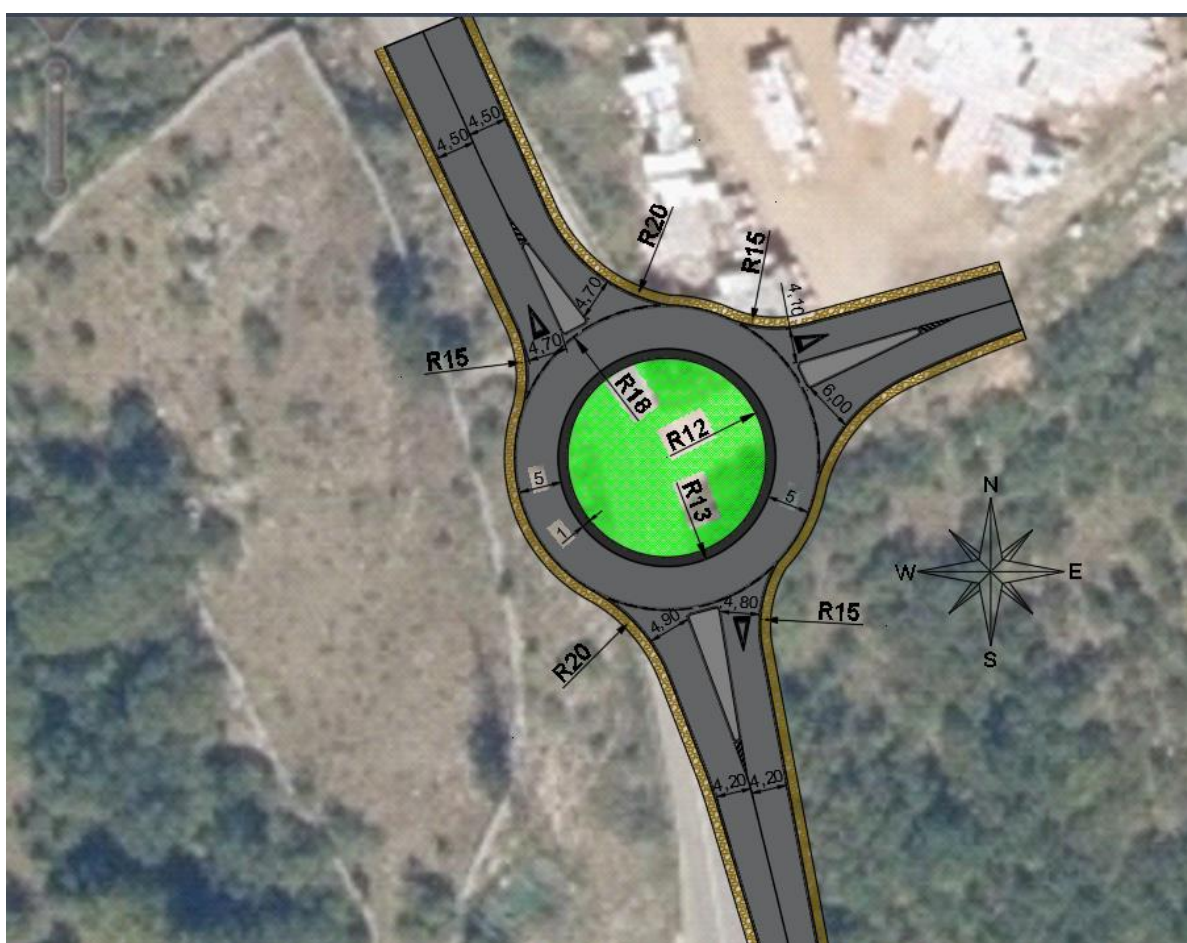
Slika 37: Kružni tok u prostoru (izradio autor)
