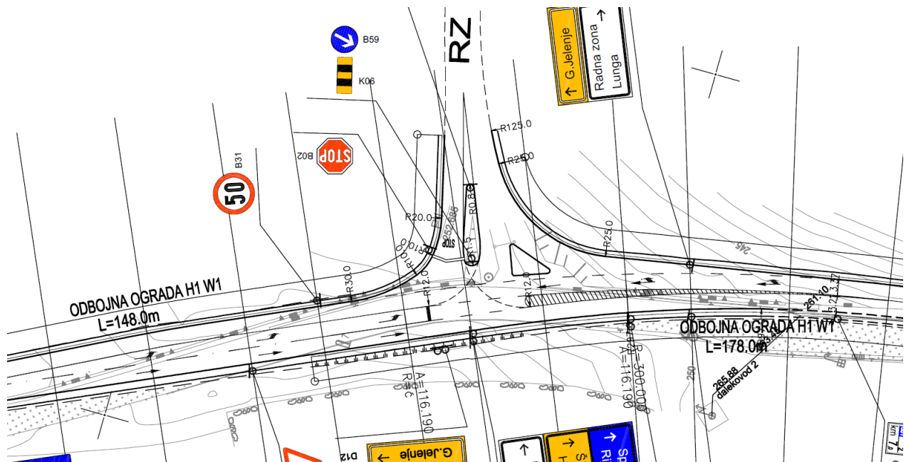
Slika 25: Prometno rješenje raskrižja za RZ Lunga [6]
