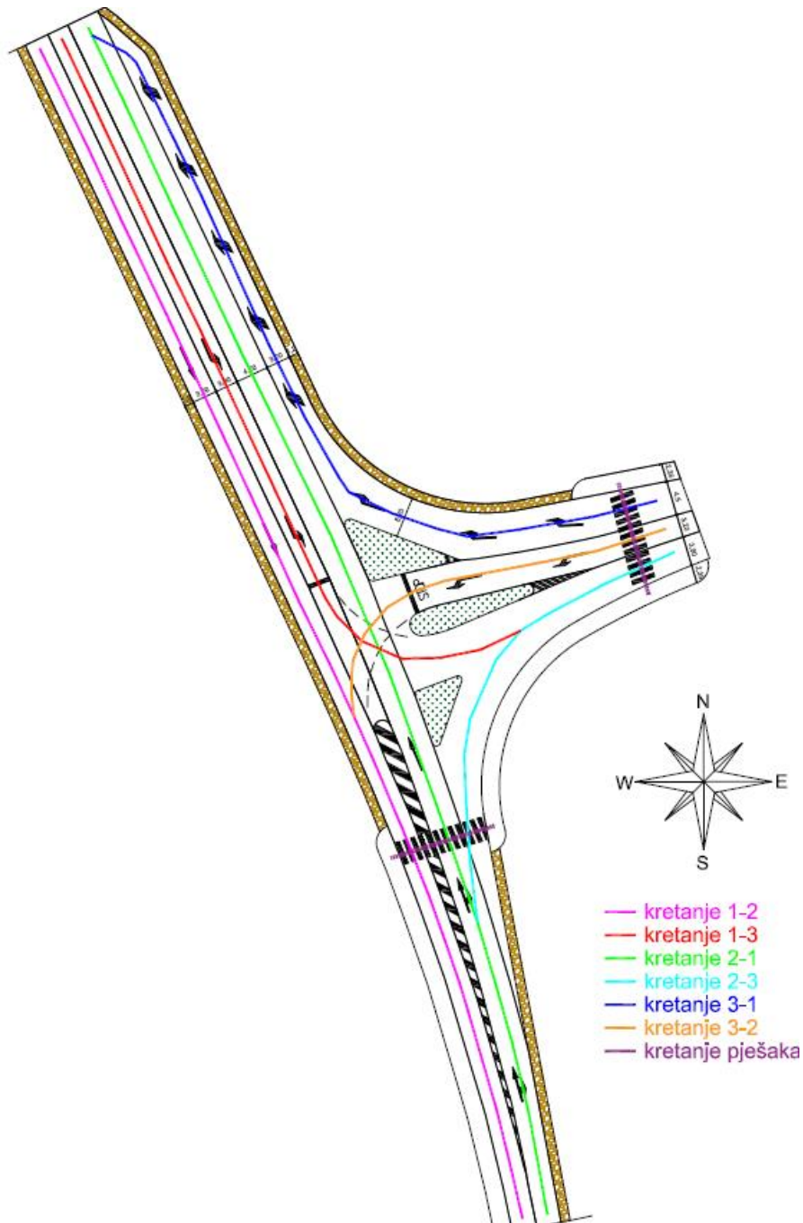
Slika 47: Smjerovi kretanja u raskrižju varijante 2 (izradio autor)
