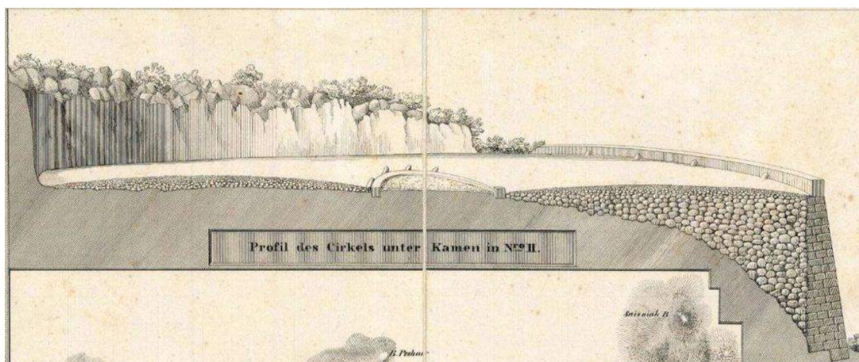
Slika 10: Profil ceste na Cirkulu kod Kamenjaka [8]
