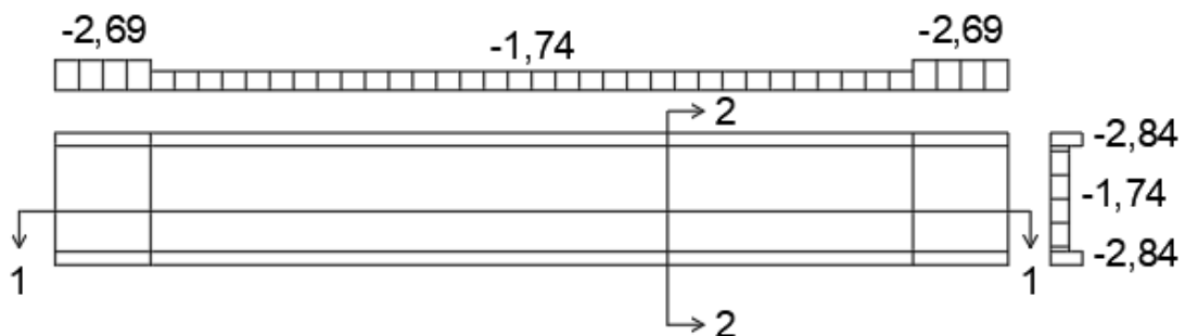
Slika 12: Opterećenje po zonama za \varphi=0^\circ
