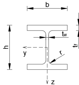
Slika 51: Skica profila HEM 1000 (stup)
