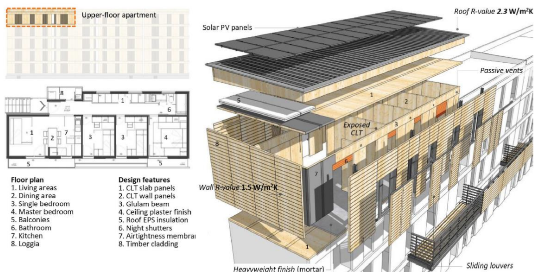
Slika 21. Tlocrt i 3D prikaz drvene pasivne zgrade u Čileu [25]
