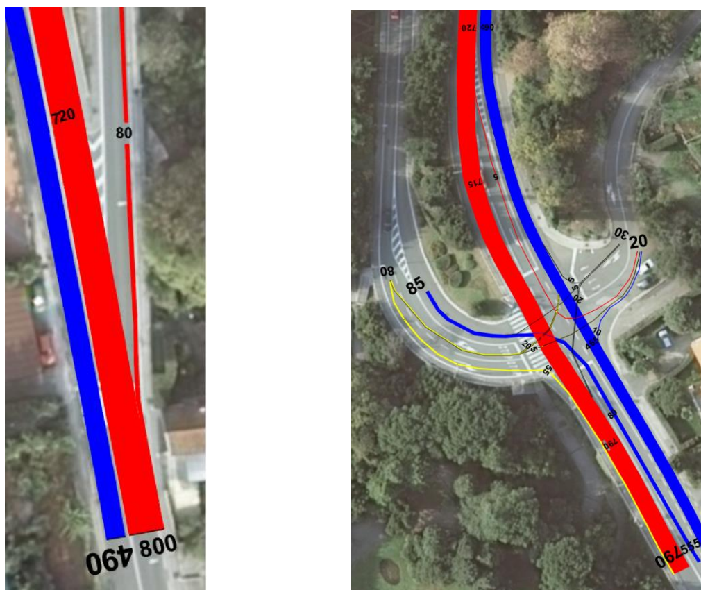
Slika 31: Prikaz pretpostavljenog grafičkog opterećenja u vršnom satu na raskrižju Vrutki
