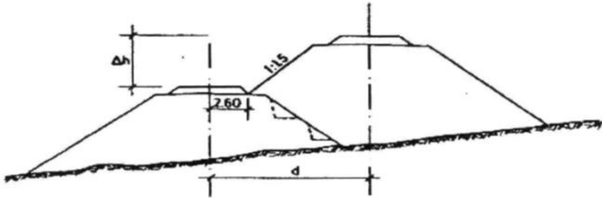
Slika 12. Veće pomjeranje kolosijeka [6]
