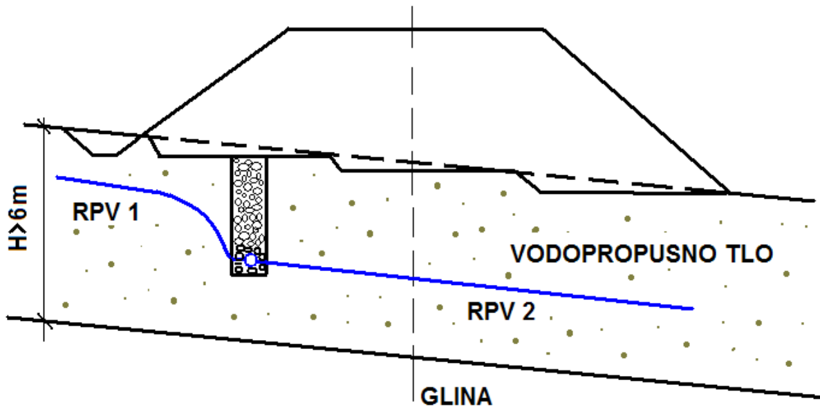
Slika 34. Duboka drenaža u slobodnoj površini [2]
