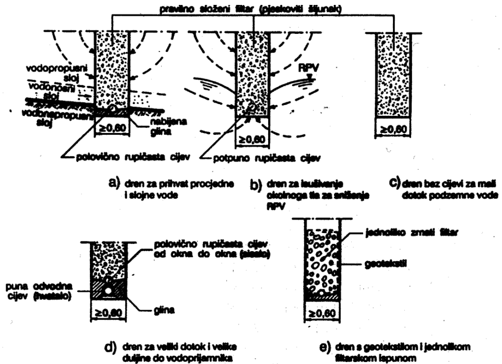
Slika 32. Vrste kopanih drenaža [8]
