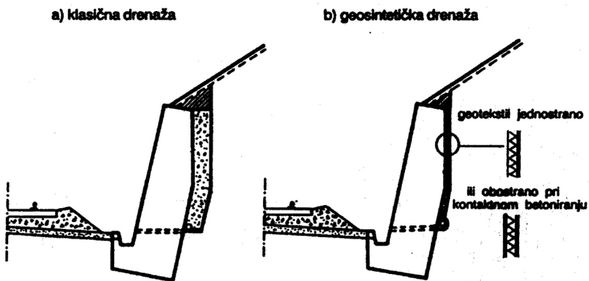
Slika 30. Usporedba klasične i geosintetičke drenaže iz zidova [8]
