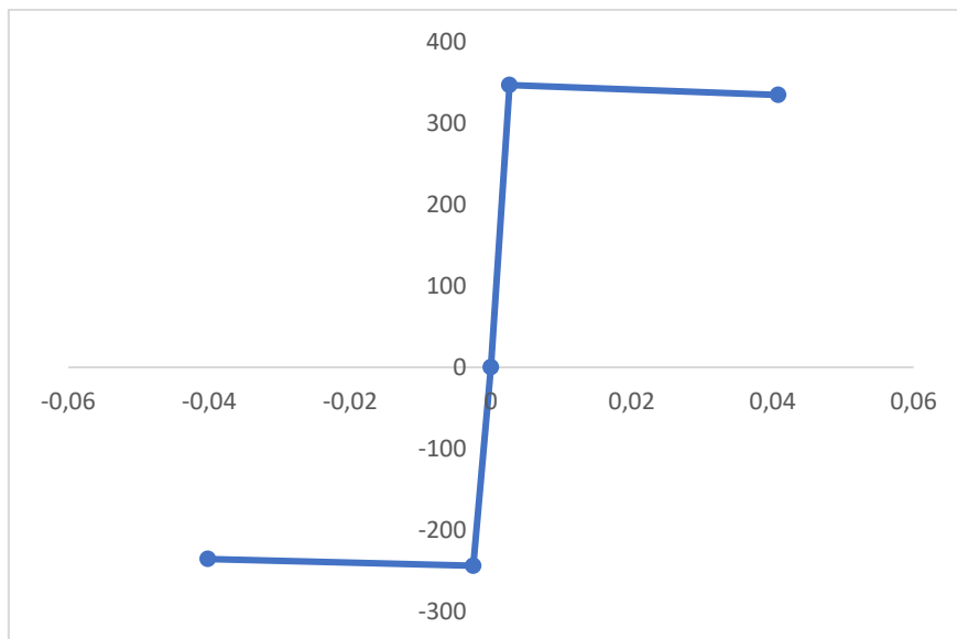
Slika 35. Dijagram M – \Theta greda 115-115 (ovijeni beton)
