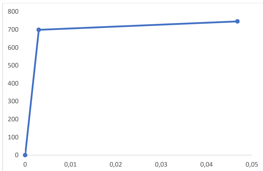
Slika 38. Dijagram M - \theta stup IV/100
