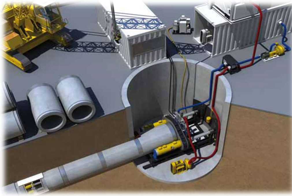
Slika 17 : Metoda mikrotuneliranja [8]
