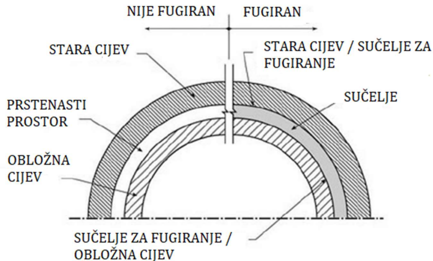
Slika 16 : Presjek cijevi kod izvođenja slip lining metode [1]
