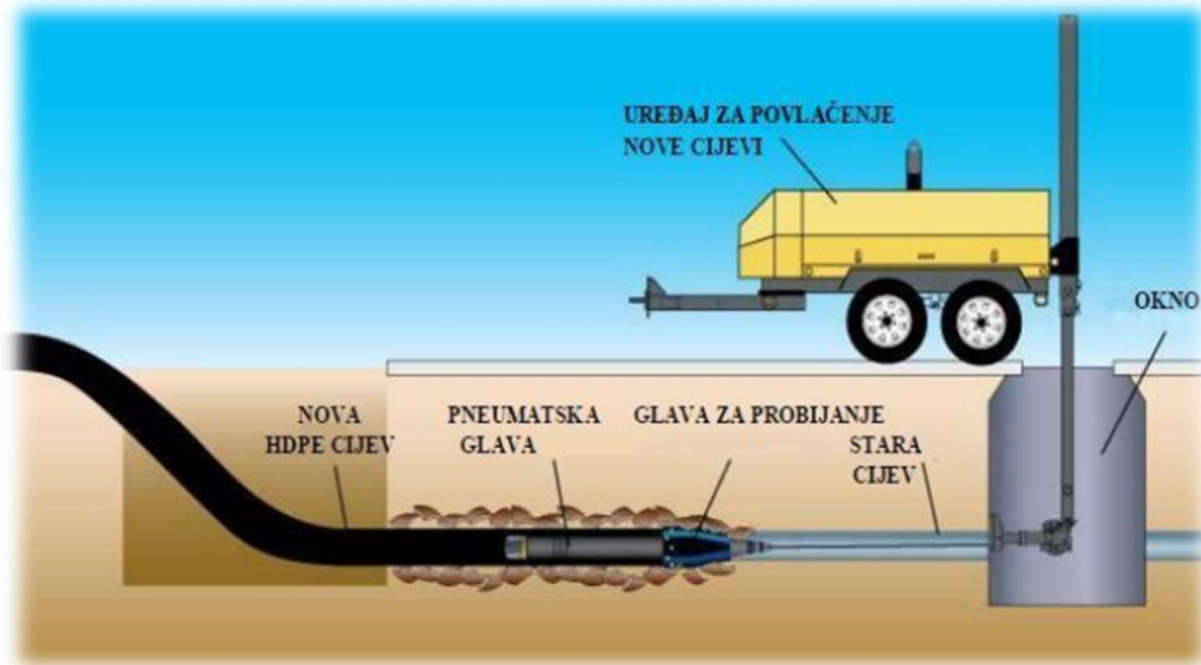
Slika 14 : Metoda proboja [5]
