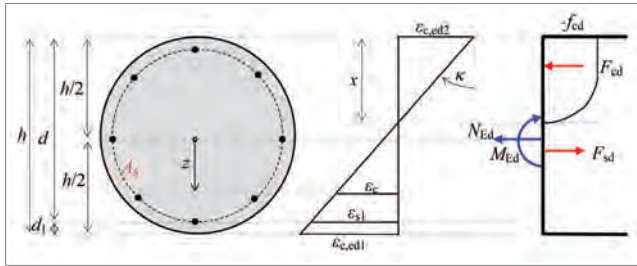
Slika 3. Kružni poprečni presjek s raspodelom naprezanja, deformacija i sile
