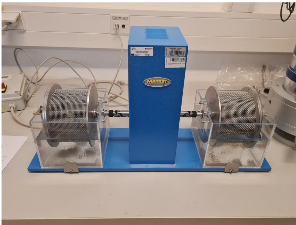
Slika 13. Uređaj za određivanje postojanosti stijene (eng. Slake Durability Test, SDT)
