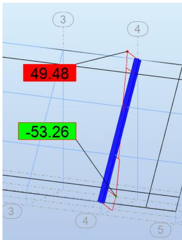
Slika 37: Poprečna sila u spoju nosača i stupa za 11. kombinaciju GSN
