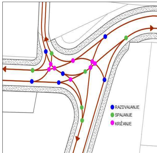
Slika 34. Konfliktne točke na raskrižju 4
