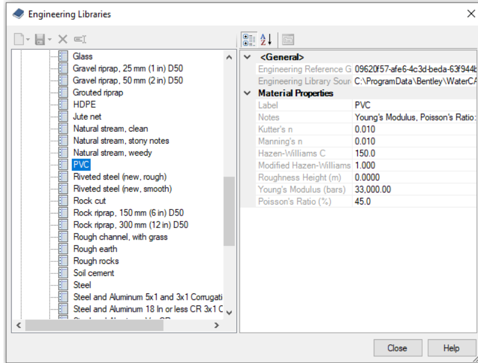
Slika 35: Karakteristike PVC cijevi unutar WaterCAD V8i računalnog programa
