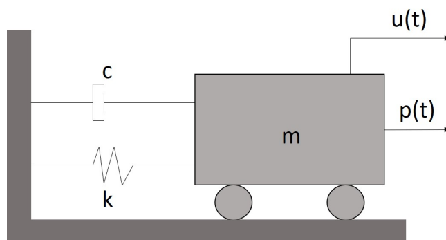
Slika 4.8: Primjer sustava s jednim stupnjem slobode
