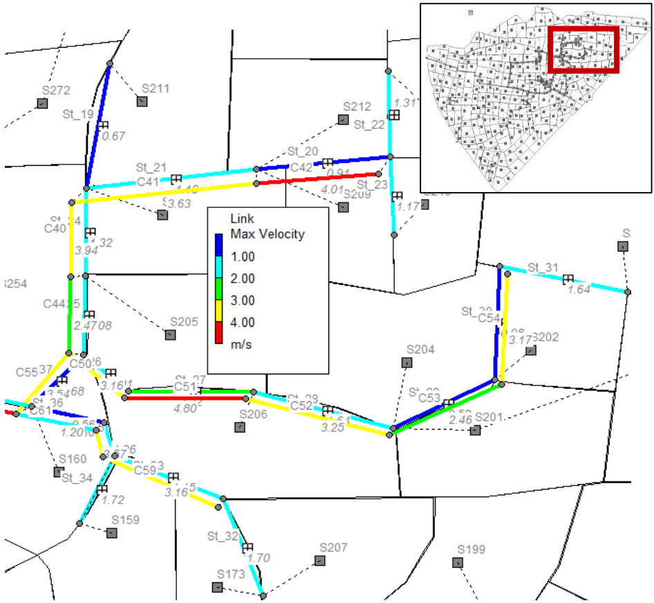
Slika 66. Grafički prikaz maksimalnih brzina u cijevima u podstavu 1 za sadašnje stanje (PP 25.god., 3h)
