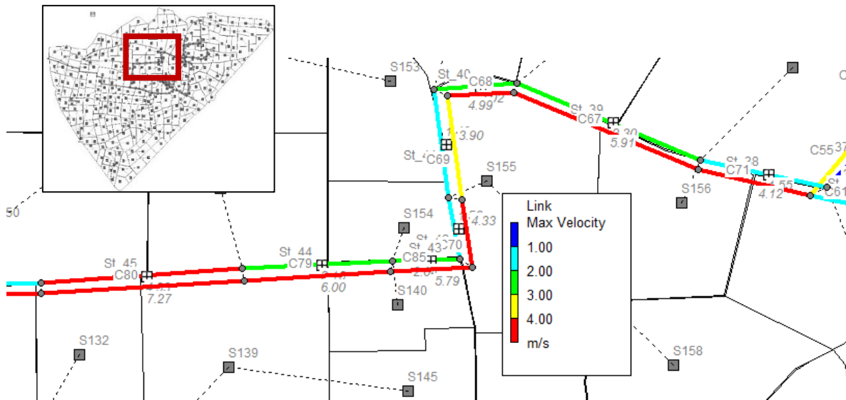
Slika 67. Grafički prikaz maksimalnih brzina u cijevima u podstavu 2 za sadašnje stanje (PP 25.god., 3h)
