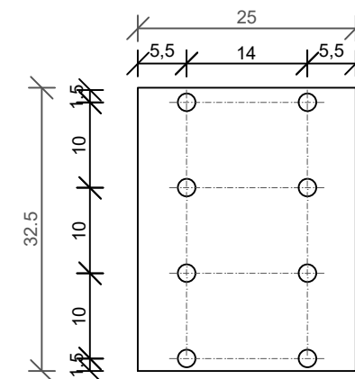
Čelična ploča S235 M=1:5
